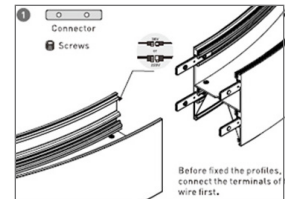
פרט חיבור
