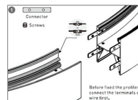
פרט חיבור
